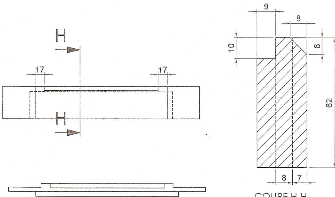
COUPE H-H ECHELLE 1 : 1
