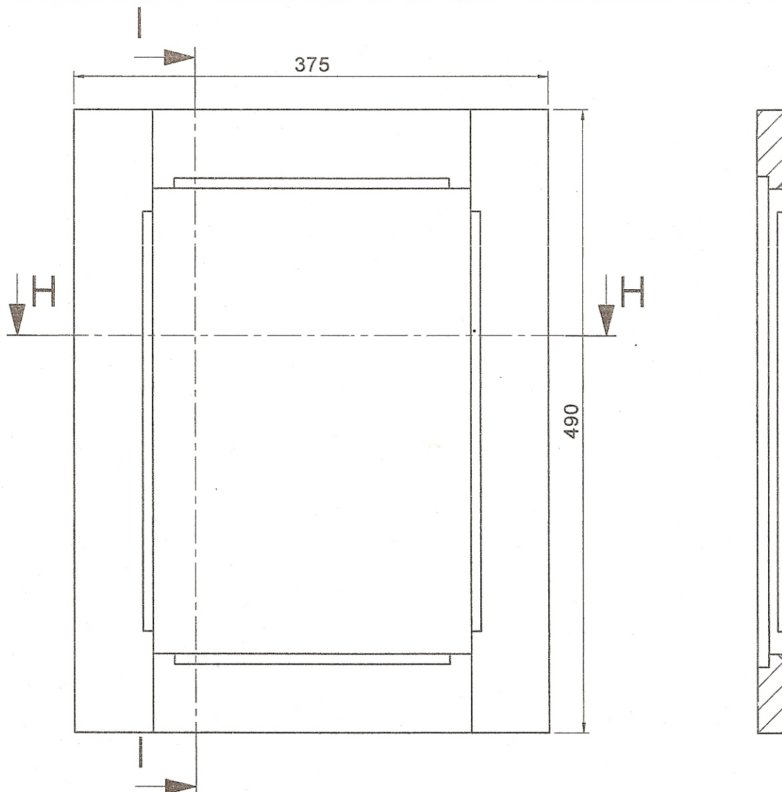
COUPE H-H ECHELLE 1 : 4
