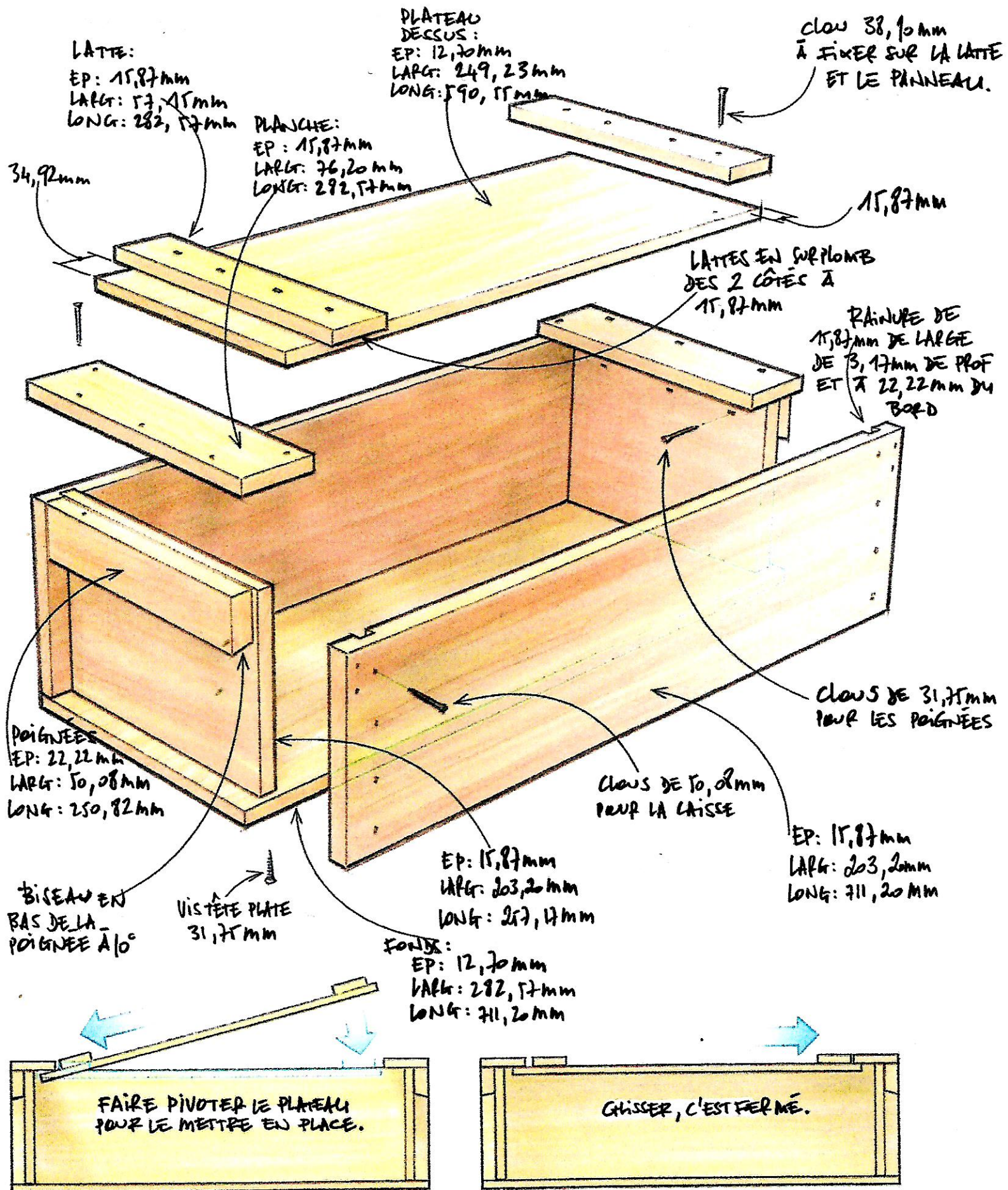
JAPANESE TOOL BOX PLAN... PLAN CAISSE À OUTILS JAPONAISE...
